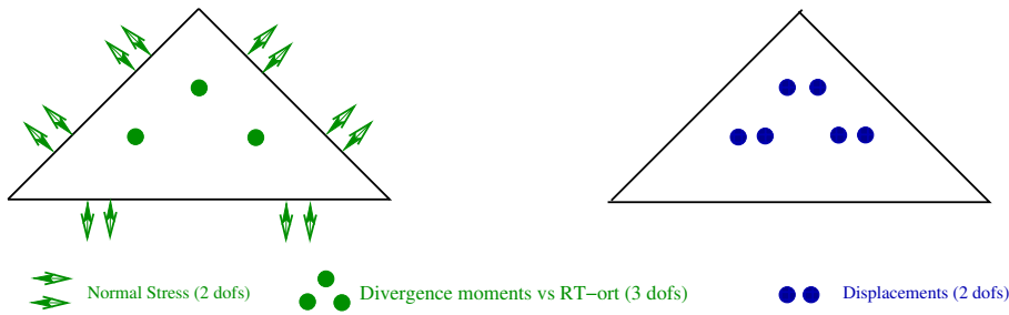
Fig. 19 Hellinger-Reissner Dofs for k = 1 , VEM HR-Virtual-VEM [11]
